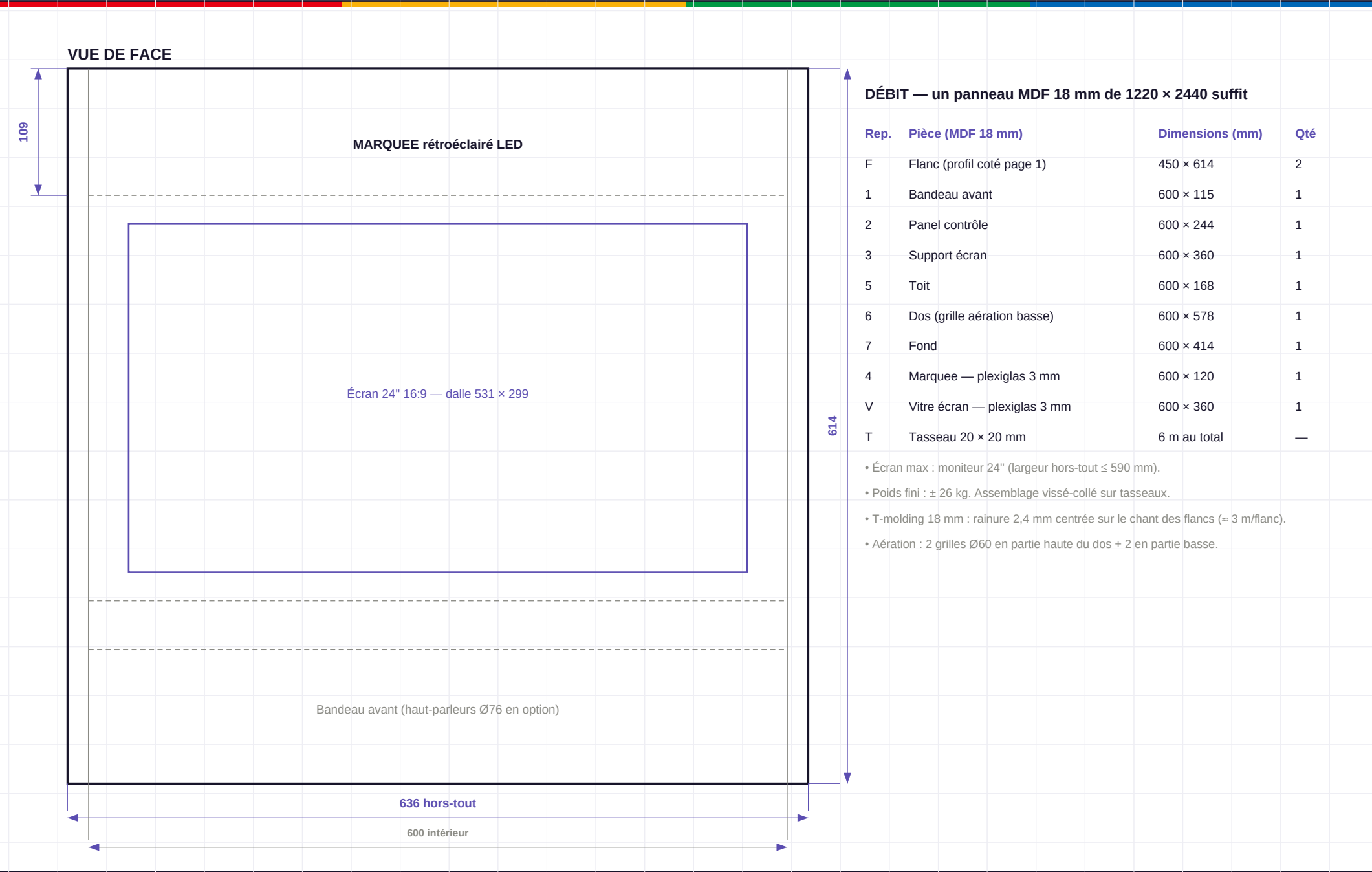
Pian bartop arcade 2 joueurs — vue de face et débit
